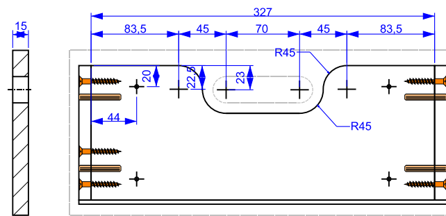
Teil Nr. 7.3 Schubkasten Boden
