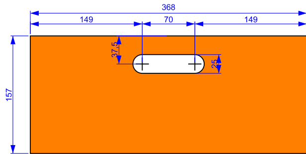
Teil Nr. 7 Schubkastenblende
