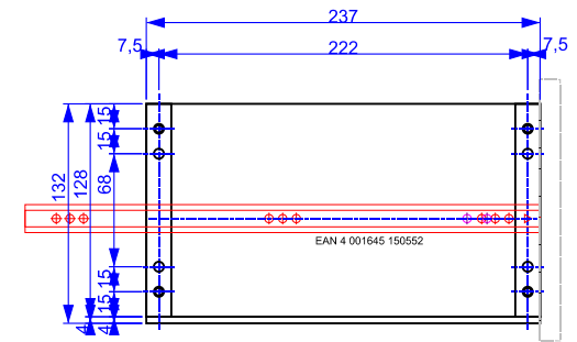
Teil Nr. 7.2 Schubkasten Seitenteil
