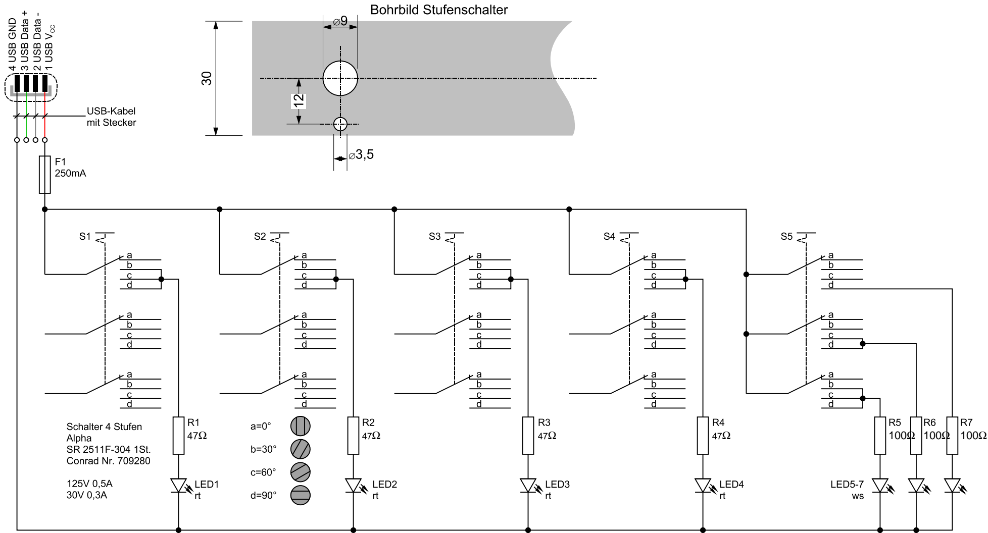
Kontroll-LEDs Herdplatten
