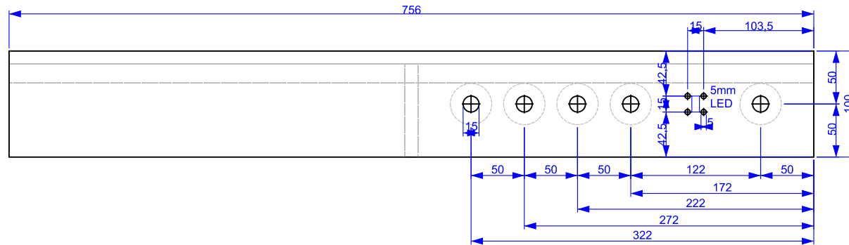
Teil Nr. ... Leiste zur Befestigung der Frontblende
