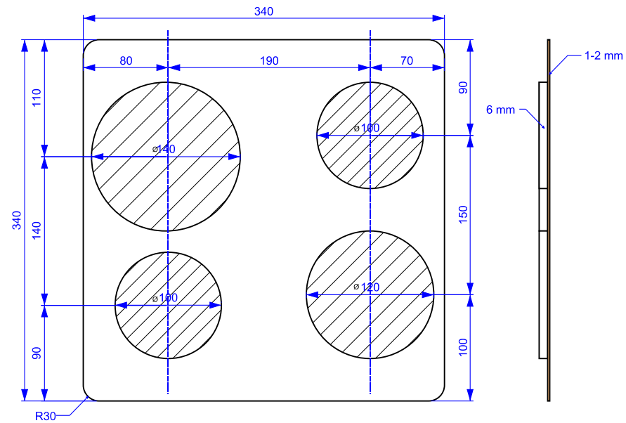
Teil Nr. 11 Kochfeld
